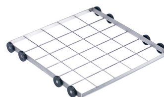
Underkurv U 876 Lafette i rustfrit stål. Placeres i stedet for U 890. Kan anvendes til alle U 500 kurve, maksimal højde på service, ved brug af O 885, er 230 mm.
