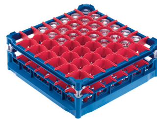
Glaskurv U 537 , ruminddelt i 7 x 7 rum til glas Ø = 63 mm, til O 885 og U 876.
