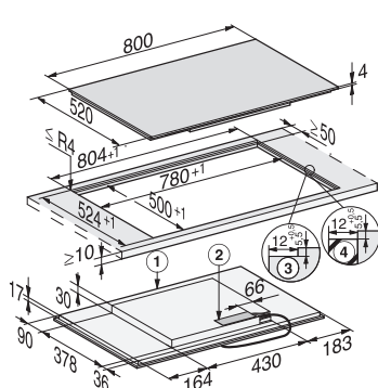
Indukčná varná doska KM 7474 FL
