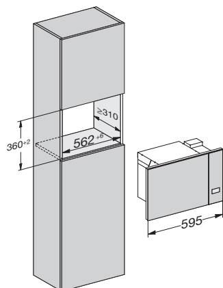
Mikrovlnná rúra M 2230/34
