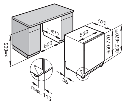
Umývačka riadu G 5350 SCVi G 5150 SCVi
