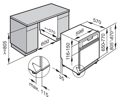
Umývačka riadu G 5310 SCi G 5110 SCi
