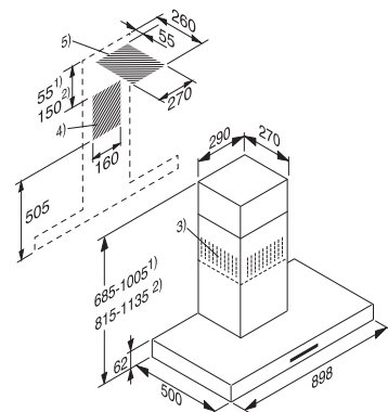
Nástenný odsávač pár PUR 98 W
