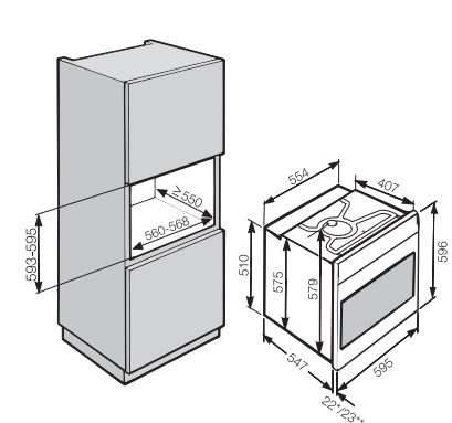
Zabudovateľná rúra na pečenie H 2465 B/BP, H 2467 B/BP, H 2861 B/BP, H 2766 B/BP
