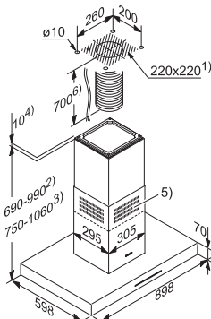
Ostrovny odsávač pár PUR 98 D
