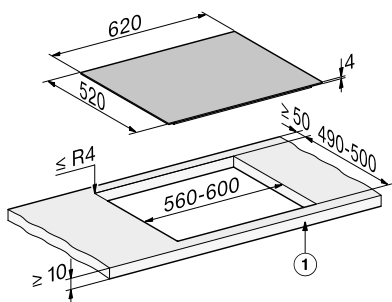
KM 7360 FL, KM 7361 FL, KM 7363 FL e KM 8462 FL Instalação sobre a bancada
