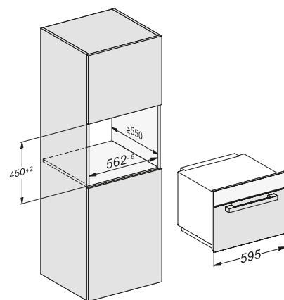
M 7140 TC M, M 7240 TC e M 7244 TC
