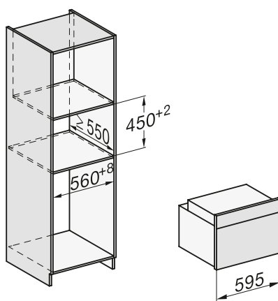
Esquema geral para fornos compactos
