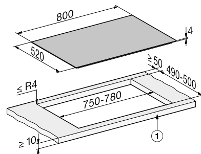
KM 7373 FL e KM 8484 FL Instalação sobre a bancada
