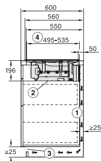
KMDA 7272 FL, KMDA 7473 FL Instalação sobre bancada, sem moldura
