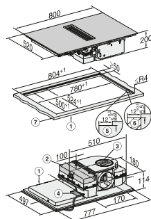
KMDA 7272 FL Instalação à face
