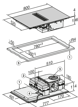
KMDA 7272 FL Instalação sobre a bancada
