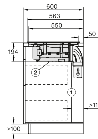
KMDA 7272 FL Instalação sobre a bancada. Instalação com saída guiada (não inclui tubos)
