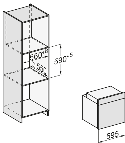
Esquema geral de encastre para fornos
