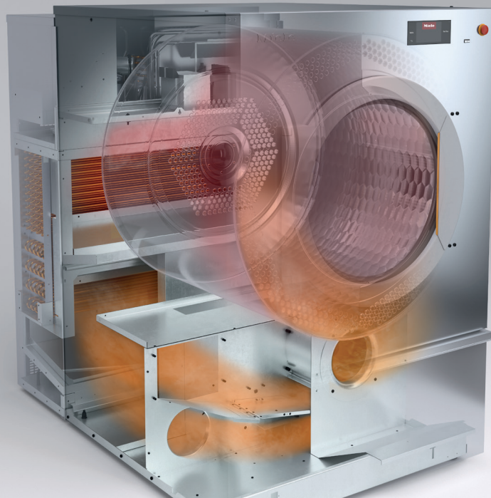
Functie warmtepompdrogers
