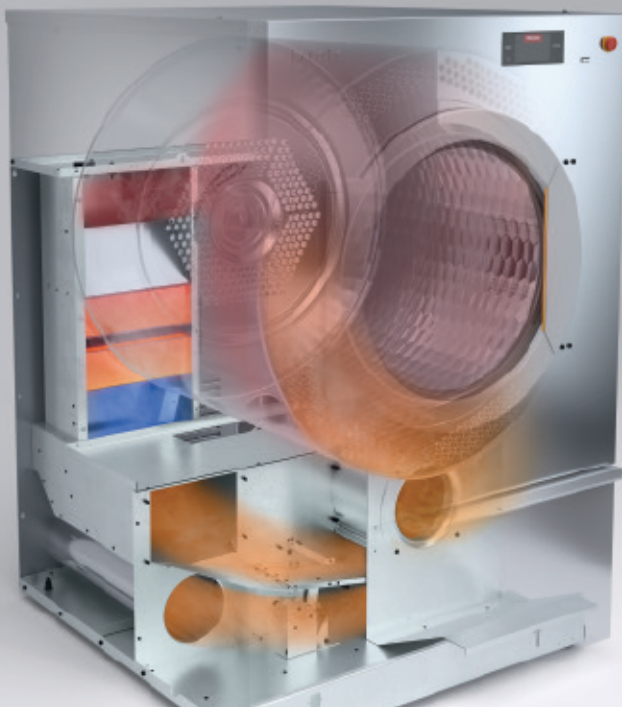
Σύστημα AirRecycling Flex
