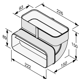
Flatkanalbend DFK-BVK 90
