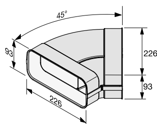
Flatkanalbend DFK-BH 45
