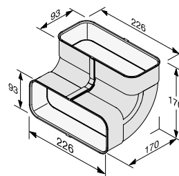
Flatkanalbend DFK-BV 90
