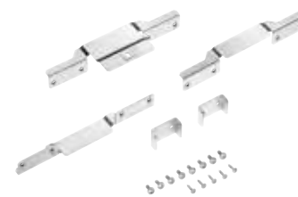
Side-by-side kit til vinskap KSK 6300
