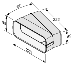
Flatkanalbend DFK-BH 15
