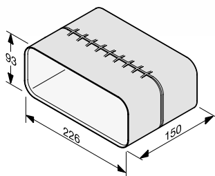
Forlenger DFK-L
