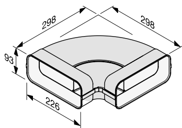
Flatkanalbend DFK-BH 90
