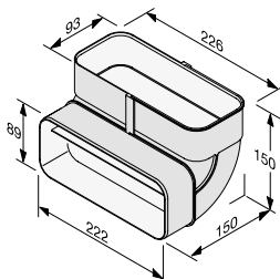
Flatkanalbend DFK-BVK 90
