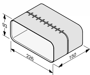
Forlenger DFK-L
