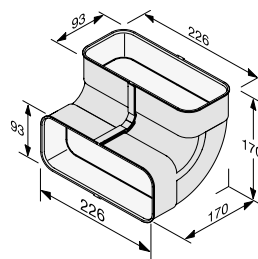
Flatkanalbend DFK-BV 90
