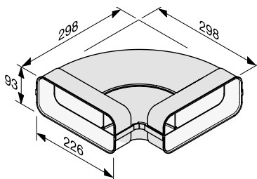
Flatkanalbend DFK-BH 90
