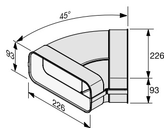
Flatkanalbend DFK-BH 45
