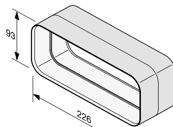
Skjøtestykke, Flatkanal DFK-V
