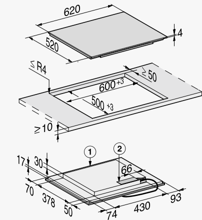
KM 7465 FL (opliggend)
