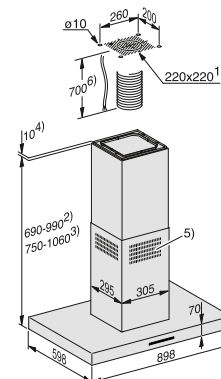
PUR 98 D, DA 4208 D / DA 4208 D EXTA
