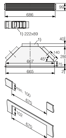
DUU 600 recirculation box
