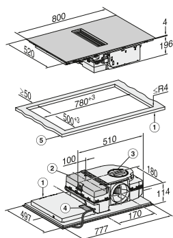
KMDA 7272 FL Montaje sobre encimera
