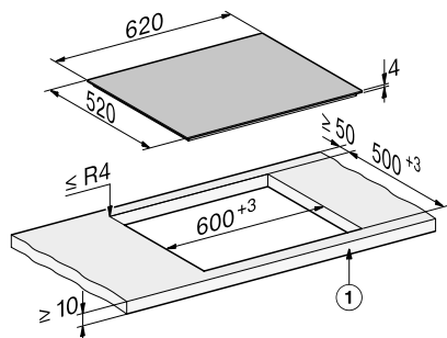
KM 8665 FL, KM 8565 FL y KM 8765 FL Instalación sobre encimera
