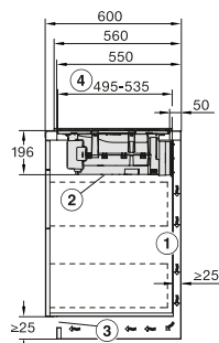
KMDA 7272 FL, KMDA 7473 FL Instalación sobre encimera, sin cerquillo
