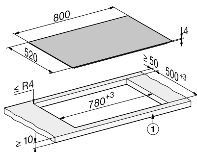
KM 8585-2FL, KM 8685-2FL y KM 8885-2FL Instalación sobre encimera
