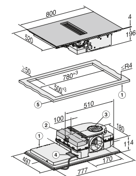
KMDA 7272 FL Montaje sobre encimera
