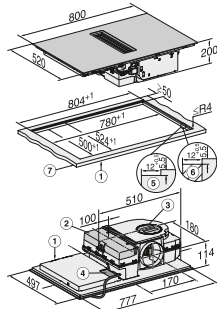
KMDA 7272 FL Montaje enrasado
