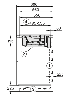
KMDA 7272 FL, KMDA 7473 FL Instalación sobre encimera, sin cerquillo
