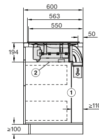
KMDA 7272 FL Montaje sobre encimera. Instalación con salida guiada (no incl. conductos)
