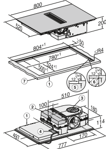
KMDA 7272 FL Montaje enrasado
