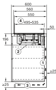
KMDA 7272 FL, KMDA 7473 FL Instalación sobre encimera, sin cerquillo
