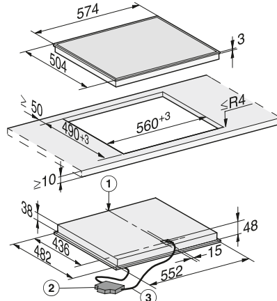
KM 6527
