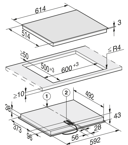
KM 6540
