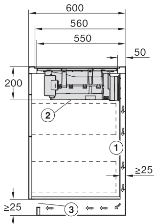
Recirculación Plug&Play
