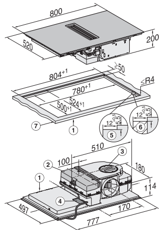
Instalación enrasada
