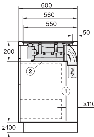
Salida de aire con conductos
