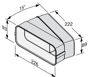
Rørbøjning 15° horizontal DFK-BH 15
