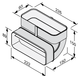
Rørbøjning 90° vertikal DFK-BVK 90
