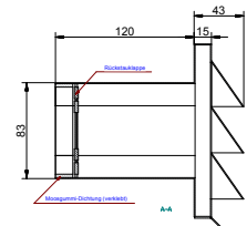
Murkasse fladkanal DFK-M
