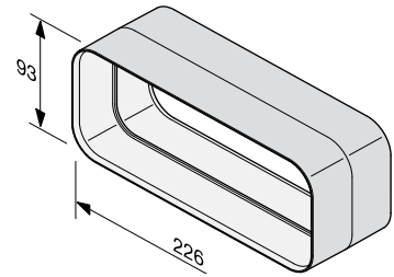
Samlestykke DFK-V
