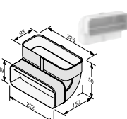
Flachkanalbogen DFK-BVK 90 M.-Nr. 10811470 IDM DFK-BVK90 45,- €*
