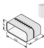
Längenausgleich DFK-L M.-Nr. 11051270 IDM DFK-L 45,- €*
