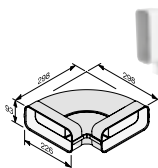
Flachkanalbogen DFK-BH 90 M.-Nr. 10811390 IDM DFK-BH90 45,- €*
