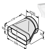
Flachkanaladapter DFK-A M.-Nr. 10811430 IDM DFK-A 45,- €*
