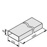
Flachkanal DFK-R 1000 M.-Nr. 10811340 IDM DFK-R1000 45,- €*
