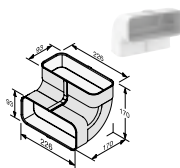
Flachkanalbogen DFK-BV 90 M.-Nr. 10811410 IDM DFK-BV90 45,- €*
