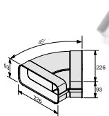
Flachkanalbogen DFK-BH 45 M.-Nr. 10811450 IDM DFK-BH45 45,- €*
