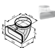
Flachkanaladapter DFK-AK 90 M.-Nr. 11590720 IDM DFK-AK90 45,- €*
