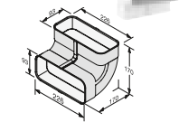
Flachkanalbogen DFK-BV 90 M.-Nr. 10811410 IDM DFK-BV90 45,- €*
