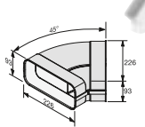
Flachkanalbogen DFK-BH 45 M.-Nr. 10811450 IDM DFK-BH45 45,- €*
