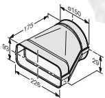
Flachkanaladapter DFK-A M.-Nr. 10811430 IDM DFK-A 45,- €*
