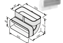
Flachkanalbogen DFK-BVK 90 M.-Nr. 10811470 IDM DFK-BVK90 45,- €*
