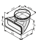
Flachkanaladapter DFK-AK 90 M.-Nr. 11590720 IDM DFK-AK90 45,- €*
