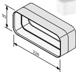
Verbindung Flach- kanal DFK-V M.-Nr. 10811360 IDM DFK-V 23,- €*
