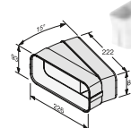
Flachkanalbogen DFK-BH 15 M.-Nr. 10811460 IDM DFK-BH15 37,- €*
