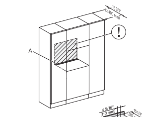
M2241SC, Einbau, 30 Zoll, Proud, breite Front – Skizze – NA
