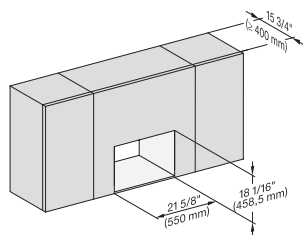
M2241SC, Einbau, 30 Zoll, Proud – Skizze – NA
