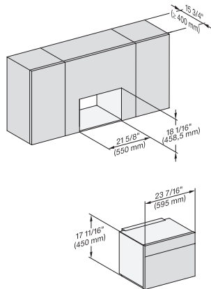
M7240TC, Einbau, 30 Zoll, Proud, breite Front, Oberschrank – Skizze – NA
