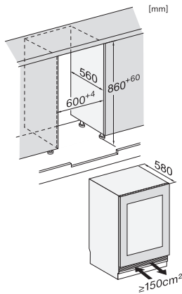
KWTUS7196E, Built-under, Einbauskizze, Nischenmaß (installation drawings)
