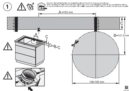
KMDA7272-1FL/FR, KMDA7473-1FL/FR, KMDA7272FL/FR, KMDA7473FL/FR, Air circulation
