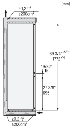
KFN7734D, KFN7734C, KFN7784D, KFN7795D, side view (US)
