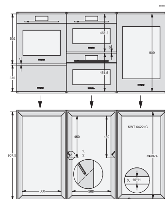
ENB1060, combination 60er & 32er EVS + 2x45er + KWT6422iG, Installation draw
