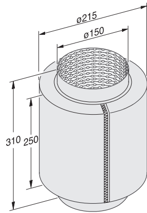
DASD150 Skizze
