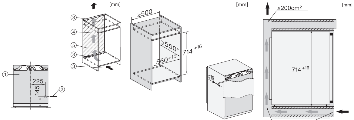
FNS7040E, FNS7040B, FNS7040C, FNS7040D, installation
