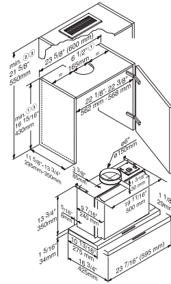
DA 3460, DA 3466 (Installation drawing) VG USA
