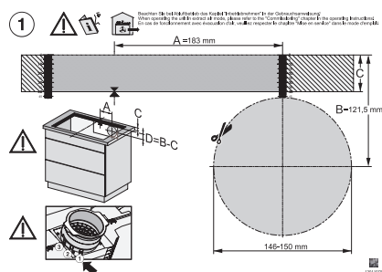
KMDA7272-1FL/FR, KMDA7473-1FL/FR, KMDA7272FL/FR, KMDA7473FL/FR, Air circulation
