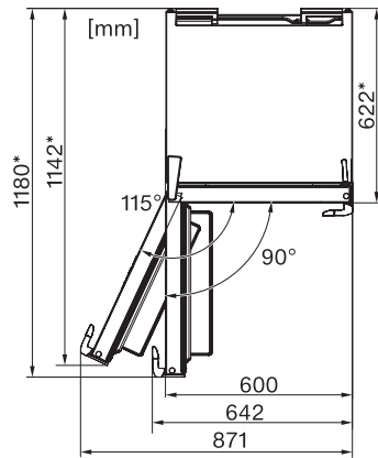
FN28262, FN28202, oppefra (skitse) (*Fodnote)
