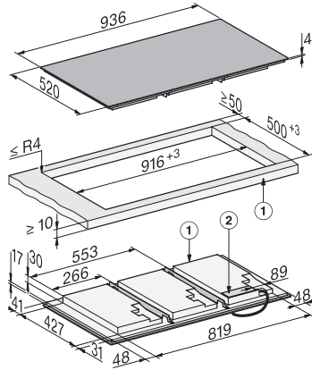
KM8695FL, KM8695FL MattFinish, aufliegender Einbau, (*Fußnote) Skizze
