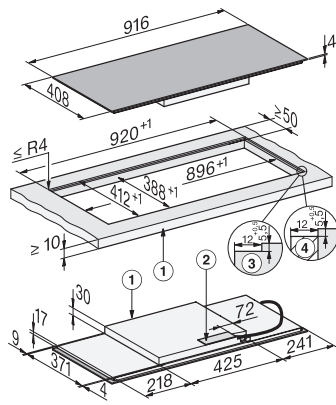
1) vorn, 2) Netzanschlusskasten, Die Netzanschlussleitung (L = 1440 mm) ist lose beigelegt, 3) Stufenfräsung Naturstein-Arbeitsplatte, 4) Holzleiste 12 mm (kein mitgeliefertes Zubehör)
