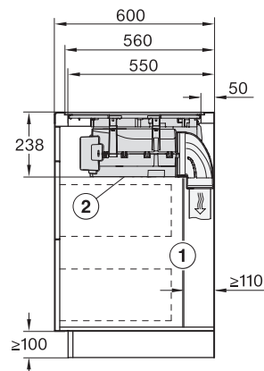
KMDA7676-1FL, KMDA7876-1FL, KMDA7676FL, KMDA7876FL – Seitenansicht flächenbündig
