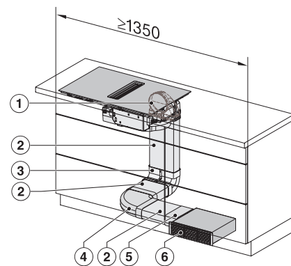
KMDA7272-1FL/FR, KMDA7473-1FL/FR, KMDA7272FL/ FR, KMDA7473FL/FR – Einbauvariante 4 Umluft
