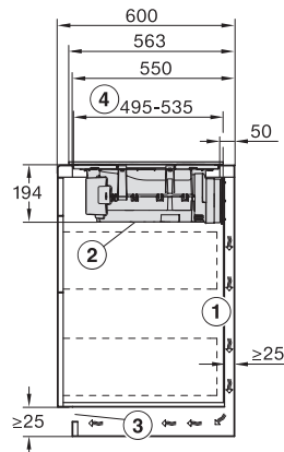
KMDA7272-1FR, KMDA7473-1FR, KMDA7272FR, KMDA7473FR – Seitenansicht aufliegend, Plug&Play
