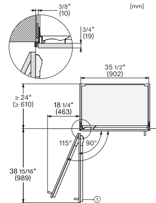
KFMC3642R, KFMC3642L, KFMC3844R, KFMC3844L, MasterCool III, PACS, mit Edelstahlfront, Draufsicht (Skizze)
