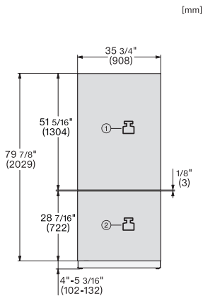
KFMC3642R, KFMC3642L, KFMC3844R, KFMC3844L, MasterCool III, Ansicht von vorne (*Fußnote) (Skizze)
