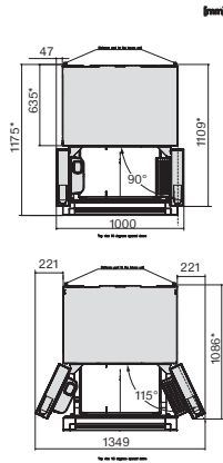
E-Com, KFFD6765 edt/cs, Draufsicht
