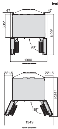
E-Com, KFFD6741 edt/cs, Draufsicht
