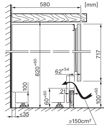
KWTUS7096E, Built-under, Seitenansicht
