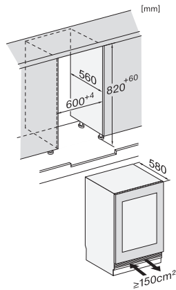
KWTUS7054F, KWTUS7055F, KWTUS7074F, KWTUS7096E, Built-under, Einbauskitze, Nischenmaß
