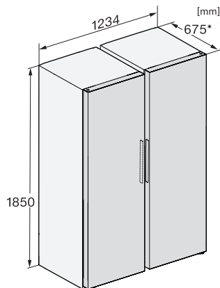
KS4383DD, KS4383ED, KS4887DD, FNS4382D, FNS4382E, FNS4882D, Aufstellskizze, Side-by-Side
