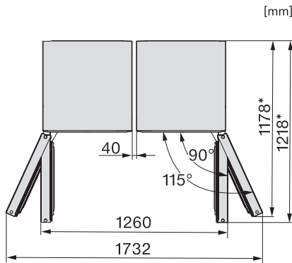
KS4383DD, KS4383ED, FNS4382E, FNS4382D, Draufsicht, Side-by-Side
