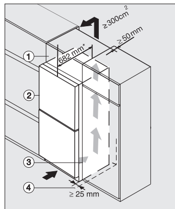
Freistehendes Kältegerät mit Glasfront in eine Küchezeile integrieren, bb, brws, bs, grgr (*Fußnote) (Skizze)
