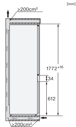
K7731F, K7731E, K7741F, Seitenansicht
