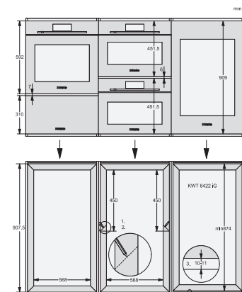
ENB1060, Kombination 60er & 32er EVS + 2x45er + KWT6422iG, Skizze
