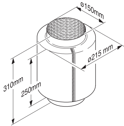
DASD150 Skizze
