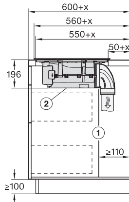
KMDA7272-1FL, KMDA7473-1FL, KMDA7272FL, KMDA7473FL – Seitenansicht aufliegend+X
