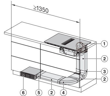
KMDA7272-1FL/FR, KMDA7473-1FL/FR, KMDA7272FL/FR, KMDA7473FL/FR – Einbauvariante 5 Umluft
