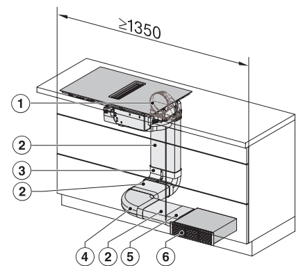
KMDA7272-1FL/FR, KMDA7473-1FL/FR, KMDA7272FL/FR, KMDA7473FL/FR – Einbauvariante 4 Umluft
