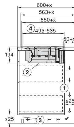
KMDA7272-1FR, KMDA7473-1FR, KMDA7272FR, KMDA7473FR – Seitenansicht aufliegend+X, Plug&Play
