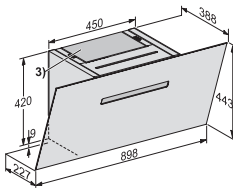
DAH1950 Skizze
