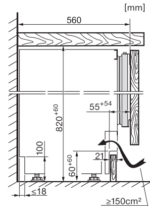
KU7016D, KU7015D, KU7035D, FNUS7040D, Built-under, Seitenansicht (Skizze)
