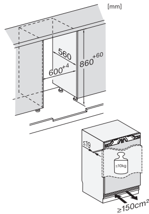
KU7135C, FNUS7140C, Built-under, Einbauskizze, Nischenmaß (Skizze)
