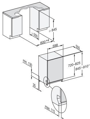
G7000 XXL, vollintegrierbare G, 60cm (Skizze), FrontFit
