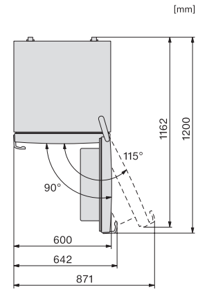
KF4472CD, Draufsicht (Skizze)
