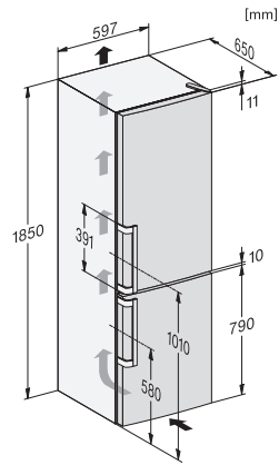
KF4472CD, Aufstellskizze (Skizze)
