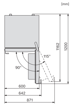
KF4472CD, Draufsicht
