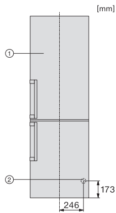
KF4472CD, Anschlusskizze
