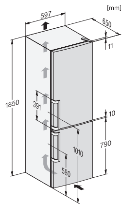
KF4472CD, Aufstellskizze
