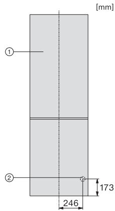
KF4372CD, Anschlusskizze (*Fußnote) (Skizze)
