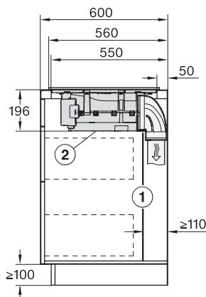
KMDA7272-1FL, KMDA7473-1FL/FL MattFinish, KMDA7272FL, KMDA7473FL – Seitenansicht aufliegend
