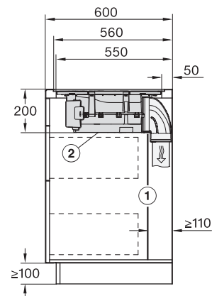
KMDA7272-1FL, KMDA7473-1FL/FL MattFinish, KMDA7272FL, KMDA7473FL – Seitenansicht flächenbündig
