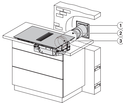
KMDA7473-1FL, KMDA7473-1FL MattFinish – Einbauvariante 15 Abluft
