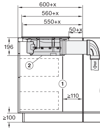
KMDA7473-1FL, KMDA7473-1FL MattFinish – Seitenansicht aufliegend+X
