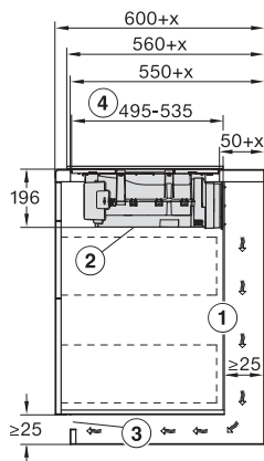
KMDA7272-1FL, KMDA7473-1FL/FL MattFinish, KMDA7272FL, KMDA7473FL – Seitenansicht aufliegend+X, Plug&Play
