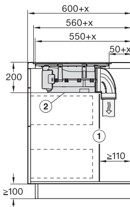
KMDA7272-1FL, KMDA 7473-1 FL/FL MattFinish, KMDA7272FL, KMDA7473FL – Seitenansicht flächenbündig+X
