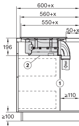
KMDA7272-1FL, KMDA7473-1FL/FL MattFinish, KMDA7272FL, KMDA7473FL – Seitenansicht aufliegend+X
